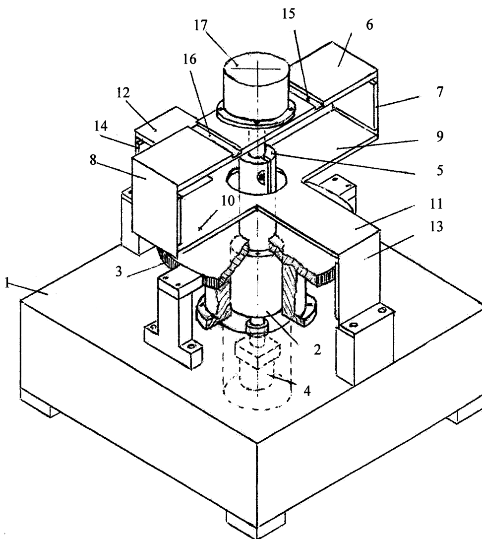
Fig. 1. kampo keitiklių kalibratorius
