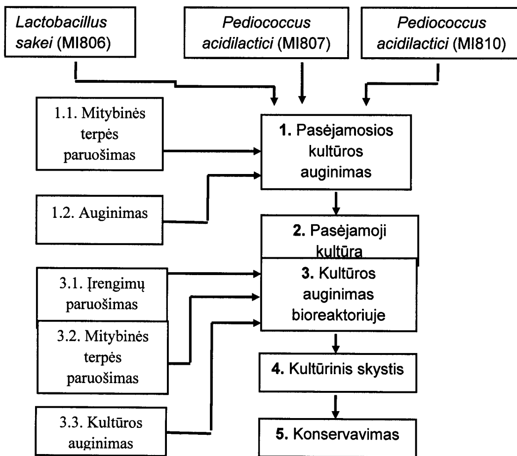
1 pav. Antimikrobinių biopreparatų fermentacijos technologinė schema (I etapas)
