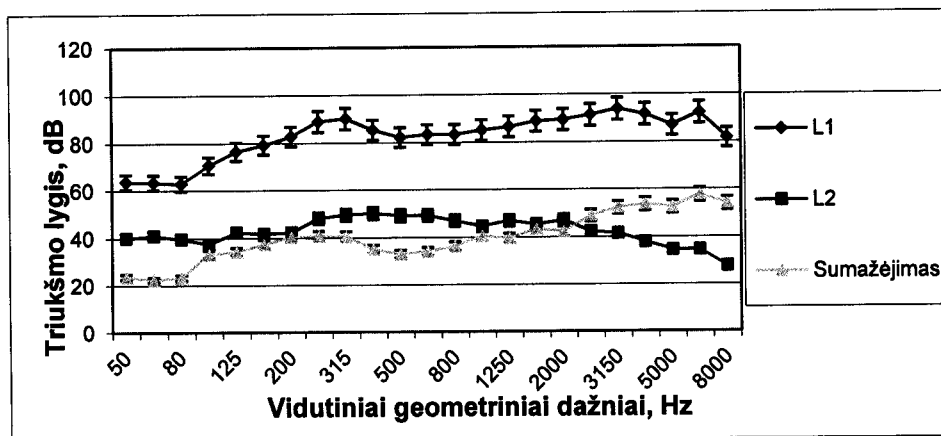
1 pav. Triukšmo lygių skirtumas. Betono ir susmulkintų padangų granulių mišinio su įgaubtu paviršiumi tyrimų rezultatai. L1 ateinantis garso lygis, L2- perėjus garso lygis
