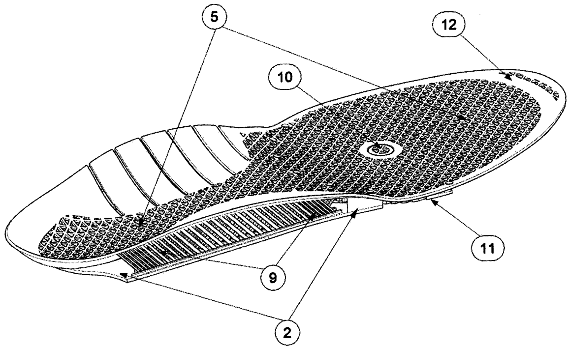
Fig. 5 Īdēklo vaizdas iš lateralinės pusės
