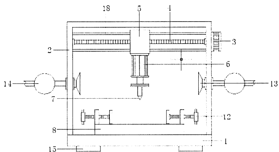
Pav. 1
