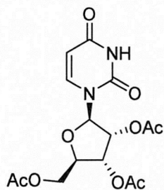
2', 3', 5'-Tri-O-acetiluridinas ( 2a )
